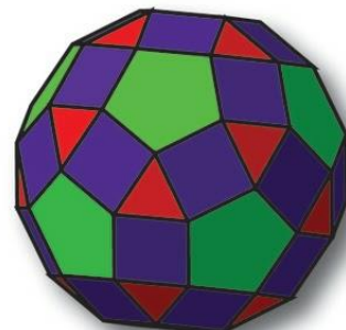
RHOMBICOSIDODECAHDRON
