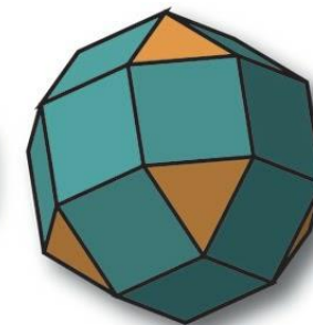
RHOMBICUBOCTOHDRON
