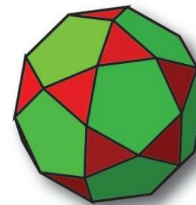
ICOSIDODECAHDRON
